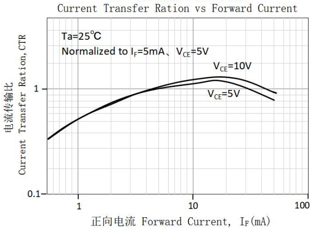
图3. 电流传输比与正向电流
