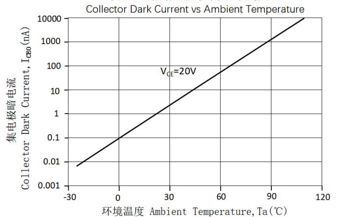
图6. 集电极暗电流与环境温度的关系
